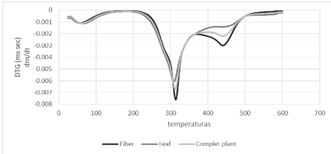
Figura 1: Curvas termogravimétricas (DTG-Mass) de Posidonia oceanica.
