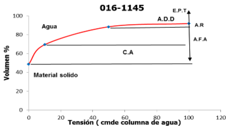
Figura 3. Curva de retención de humedad de la arena. Nota: ADD: Agua débilmente disponible, AFA: Agua fácilmente asimilable, AR: Agua de reserva.
