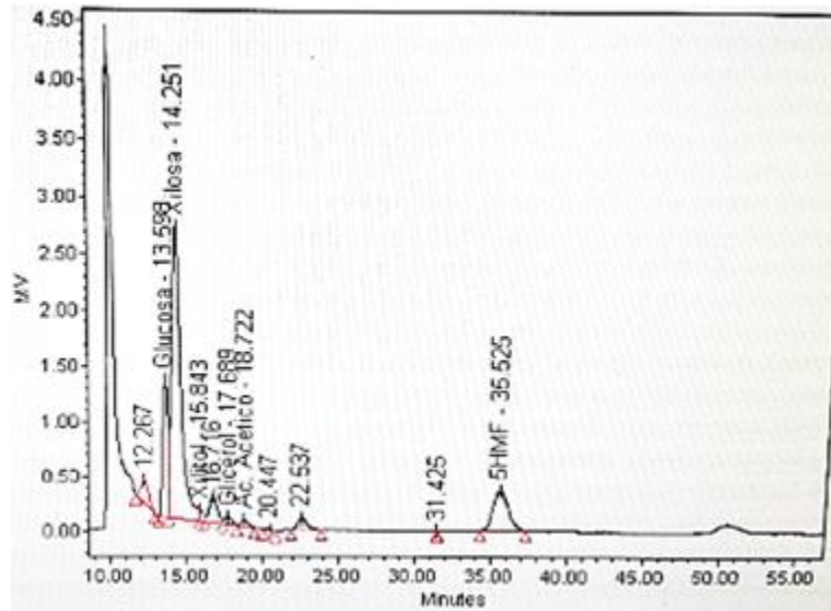
Figura 3. Perfil de carbohidratos de aserrín de P. patula autohidrolizado por steam explosión.
