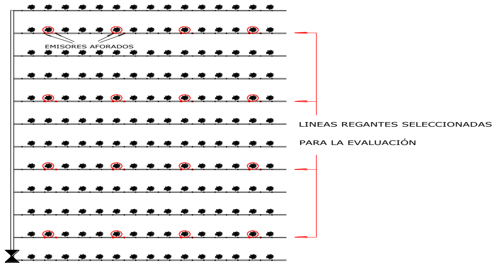
Figura 1. Líneas regantes seleccionadas para la evaluación de la unidad de riego por goteo.
