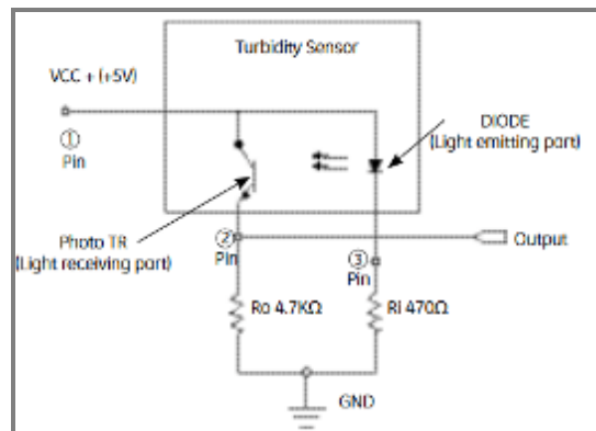
Figura 1. Circuito de acondicionamiento para el sensor.
