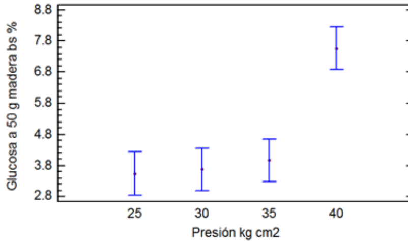
Figura 4. Gráfica de medias y 95% de Fisher (LSD) de glucosa respecto a presión de hidrólisis fisicoquímica.
