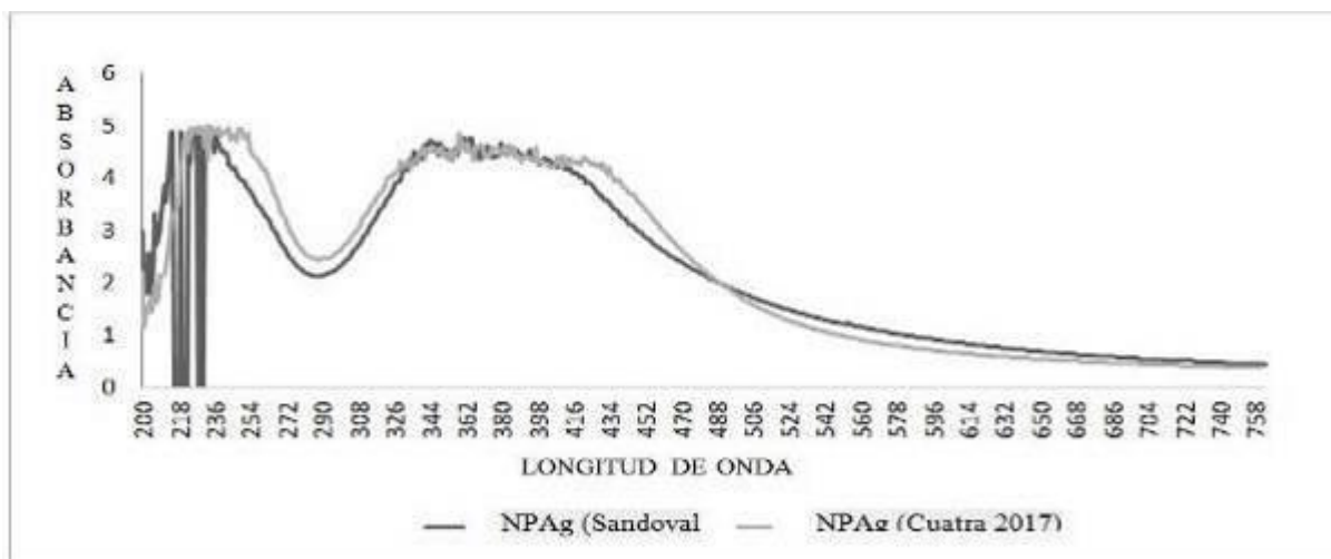
Figura 1. Espectro de absorción de las nanopartículas de plata obtenidas en la presente investigación y las obtenidas por Sandoval-Cárdenas (2012).
