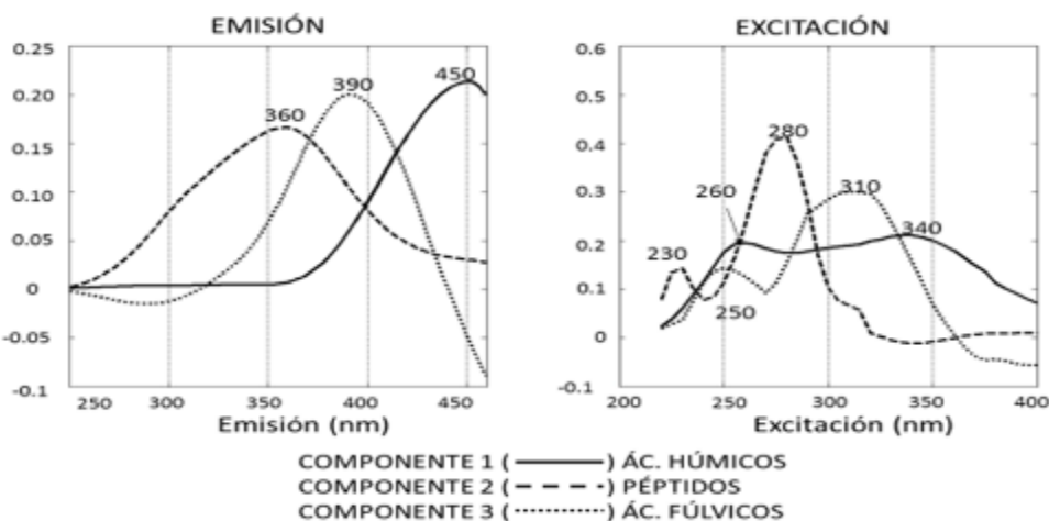
Figura 6. Representación aislada de los componentes obtenidos para el estudio de muestra de compost, señalando los picos máximos de longitud de onda de emisión y excitación. Componente 1 (ácidos húmicos), Componente 2 (péptidos) y Componente 3 (ácidos fúlvicos).
