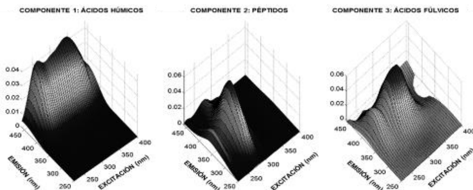
Figura 5. Representación de los componentes o fluoróforos encontrados en la muestra de compost aislada con el modelo de PARAFAC.
