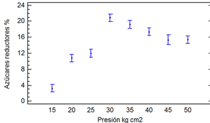
Figura 1. Gráfica de medias y 95% de Fisher (LSD) de azúcares reductores respecto a la autohidrólisis por steam explosión.
