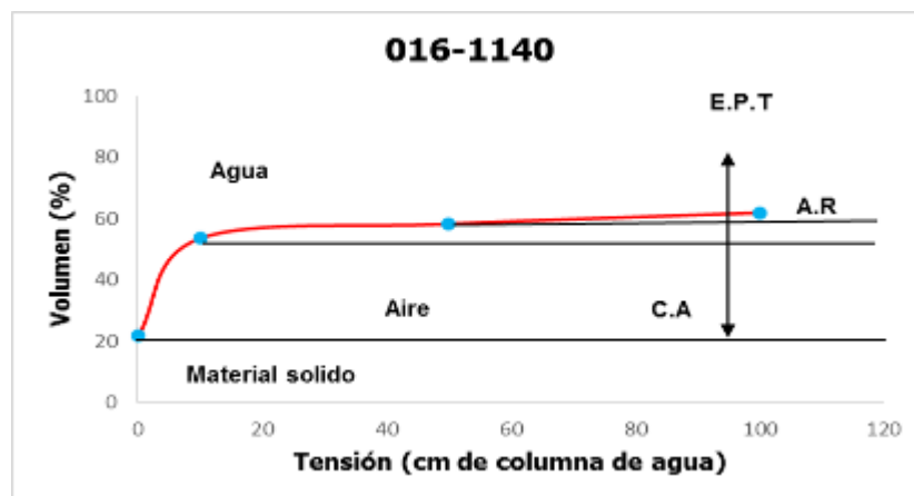
Figura 1. Curva de retención de humedad de la piedra pómez. Nota: ADD: Agua difícilmente disponible, AFA: Agua fácilmente asimilable, AR: Agua de reserva.
