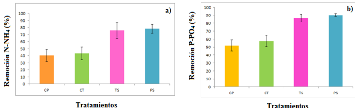
Figura 4. a) Remoción de amonio, b) remoción de fosfatos en los humedales en estudio. CP: Control piedra, CT: Control tezontle, TS: Tezontle con planta, PS: Piedra con planta.
