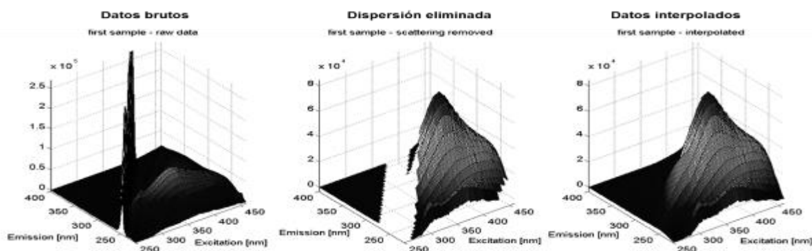
Figura 1. Espectro de EEM de los datos brutos, con dispersión eliminada e interpolada para la muestra del material inicial para compost “lodos depuradora 45”.
