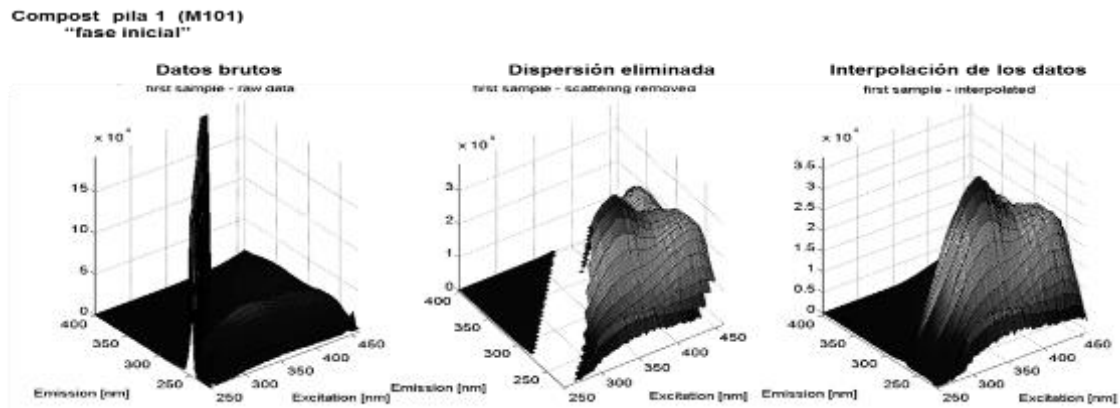
Figura 3. Espectro de EMM de los datos brutos, con dispersión eliminada e interpolada para la muestra de compost pila 1 (M101) en “fase inicial”.
