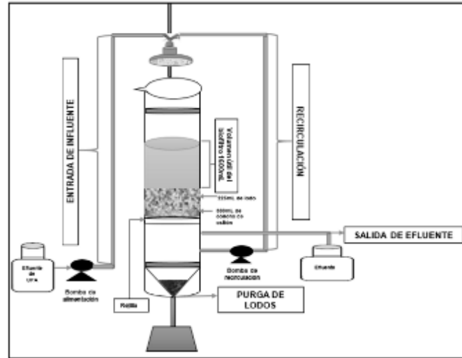
Figura1. Esquema de filtro biológico.
