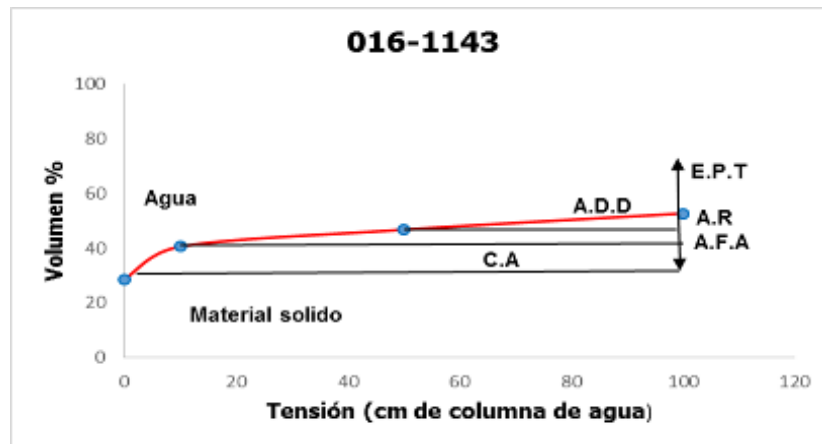
Figura 2. Curva de retención de humedad del lodo. Nota: ADD: Agua débilmente disponible, AFA: Agua fácilmente asimilable, AR: Agua de reserva.
