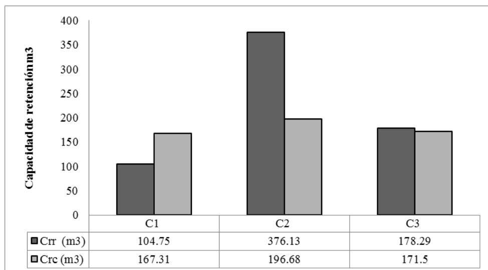
Figura 24. Capacidad real de retención de suelos (Crr) y calculada (Ccr) de las presas de morillos.
