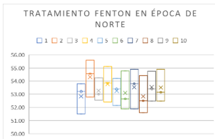
Figura 4. Resultados del tratamiento del lixiviado con reactivo Fenton en época de lluvia.
