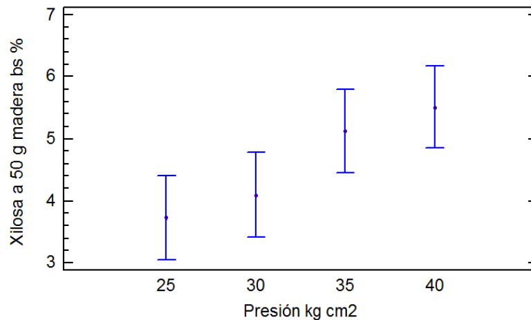
Figura 5. Gráfica de medias y 95% de Fisher (LSD) de xilosa respecto a presión de hidrólisis fisicoquímica.
