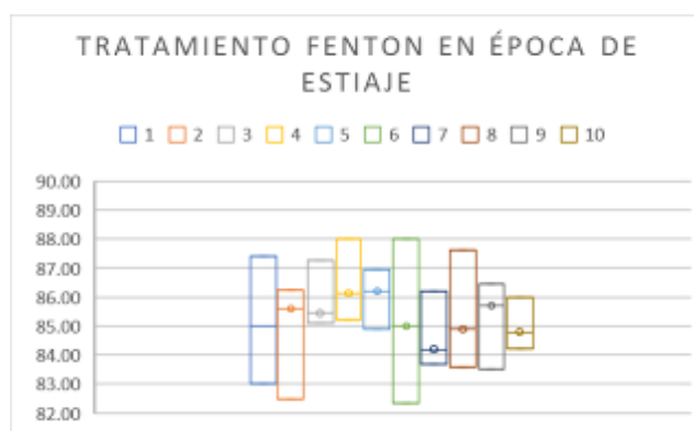
Figura 2. Resultados del tratamiento del lixiviado con reactivo Fenton en época de estiaje.
