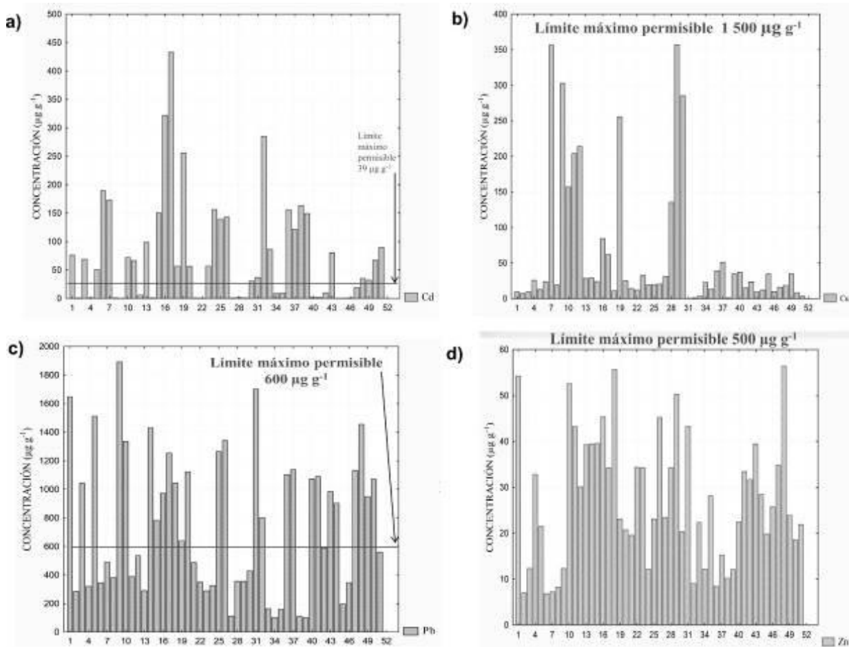
Figura 2. Concentración y límites máximos permisibles de metales pesados. a) Cd, b) Cu, c) Pb y d) Zn.
